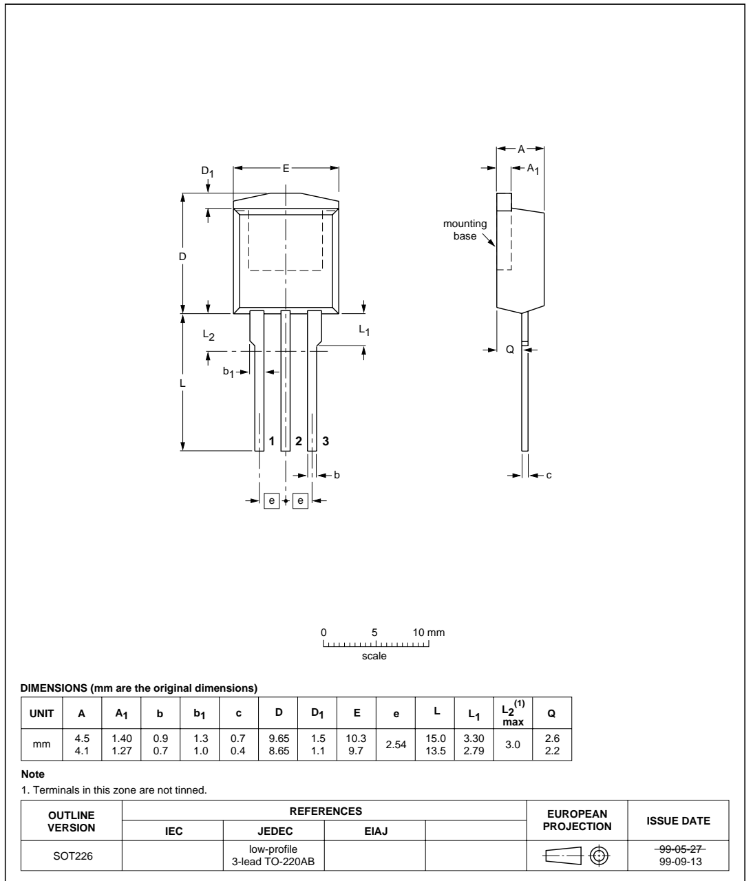
Fig.2. SOT226
